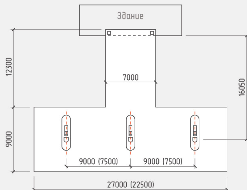
Навесная группа “Стандарт 3Т15 моноколонна”
