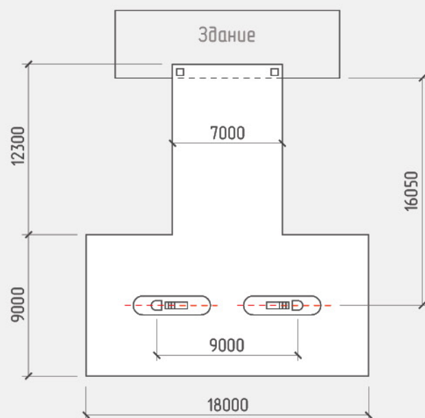
Навес над ТРК “Стандарт 2Т15 (90) моноколонна”
