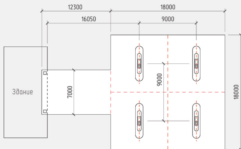
Габаритные размеры навесной группы “Стандарт (2+2)Т15”
