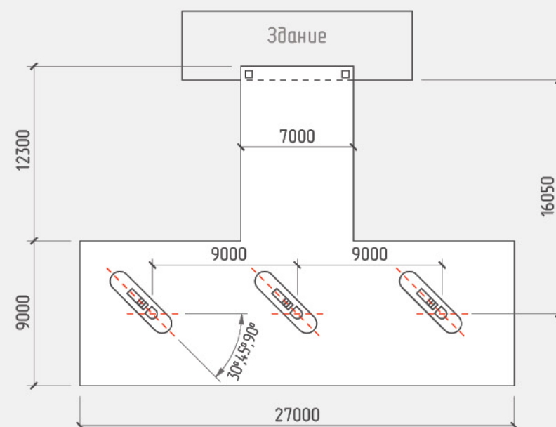
“Стандарт 3Т15 моноколонна” с поворотом колонн
