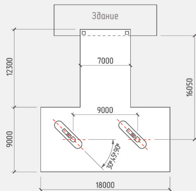
“Стандарт 2Т15 моноколонна” с поворотом колонн
