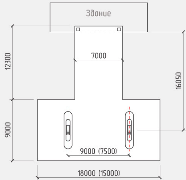
Навес над ТРК “Стандарт 2Т15”
