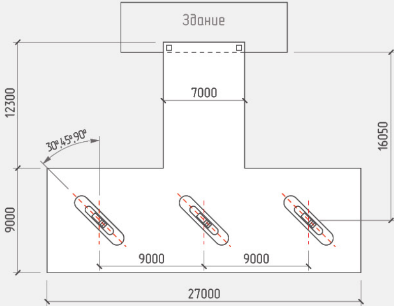
Навесная группа “Стандарт 3Т15” с поворотом колонн
