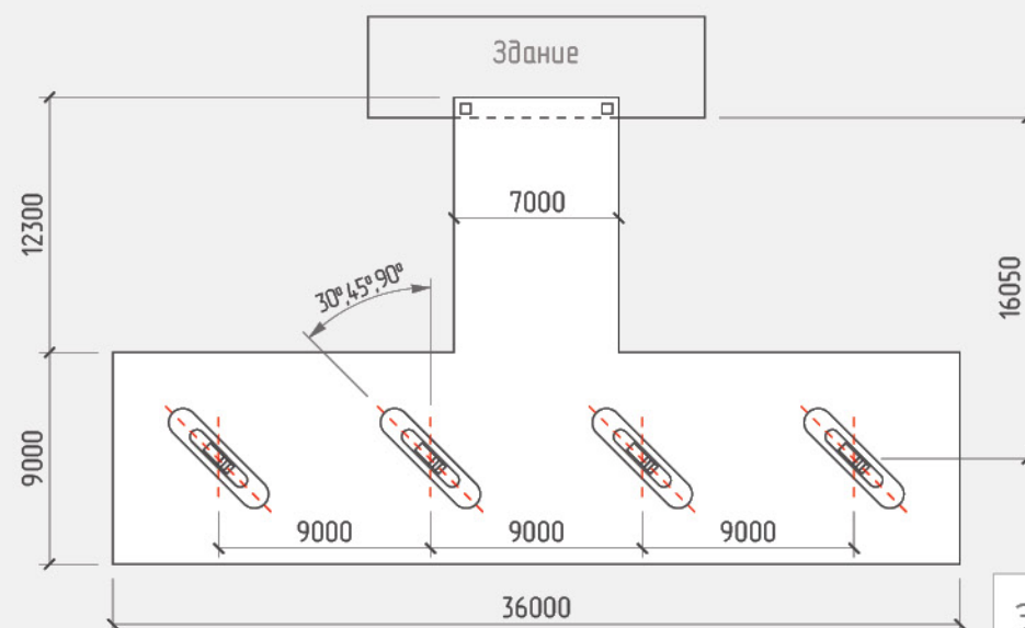
Навесная группа “Стандарт 4Т15” с поворотом колонн
