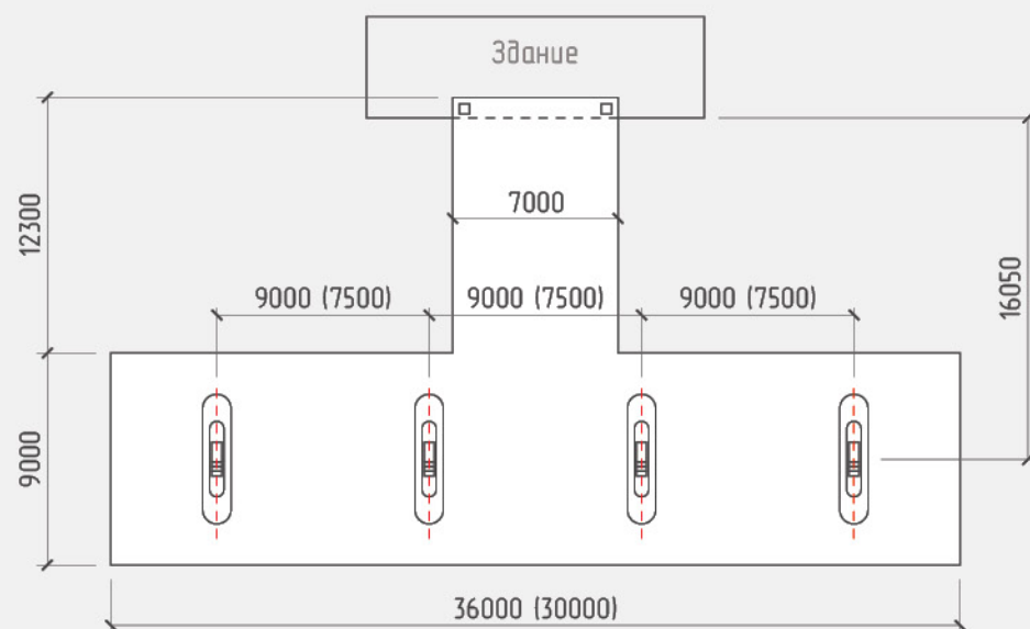
Навесная группа “Стандарт 4Т15”
