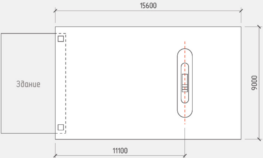
Габаритные размеры навеса над ТРК “Стандарт 1П”
