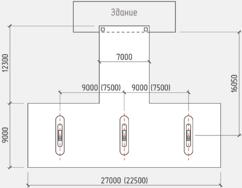
Навесная группа “Стандарт 3Т15”
