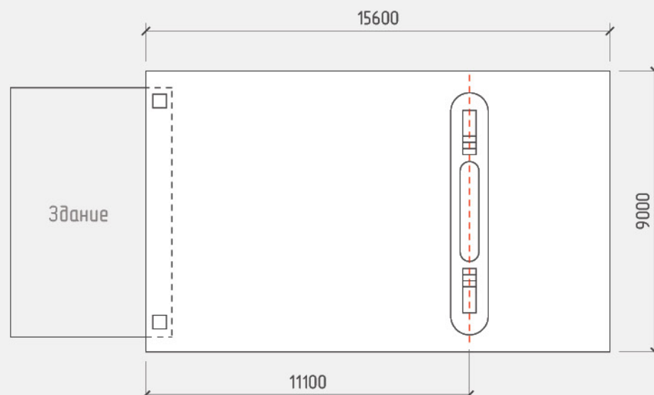
Габаритные размеры навеса над ТРК “Стандарт 1V”
