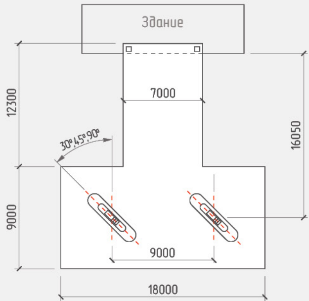
Навес над ТРК “Стандарт 2Т15” с поворотом колонн
